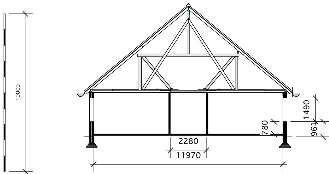
dwarsdoorsnede
